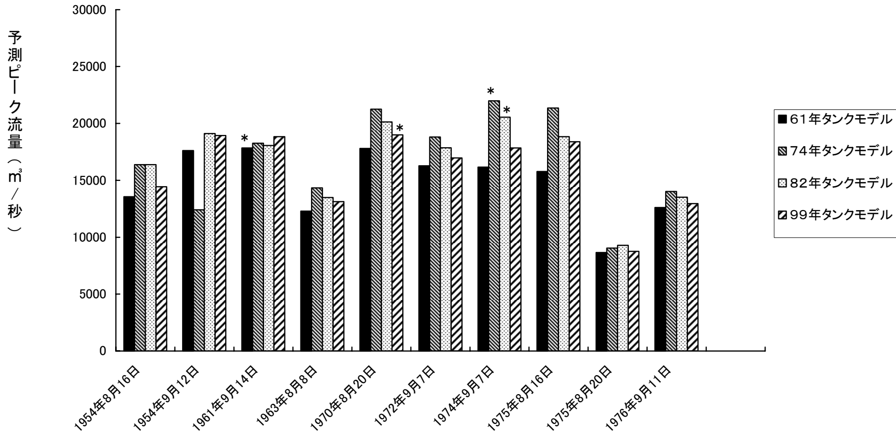
図-5 過去10回の洪水を150年に1度の洪水雨量に引き伸ばして各年度のタンクモデルで計算された基準点 (岩津)における基本高水流量(ピーク流量)
